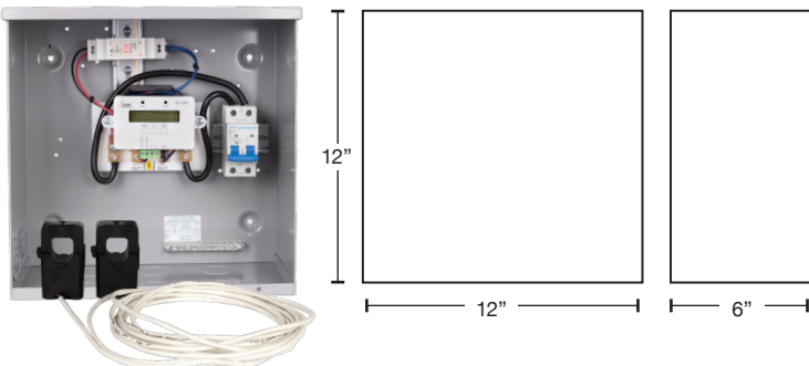
SAK-100MSB-M
